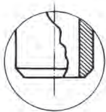
Extrémité à souder suivant ANSI B 16-25 - 2007
